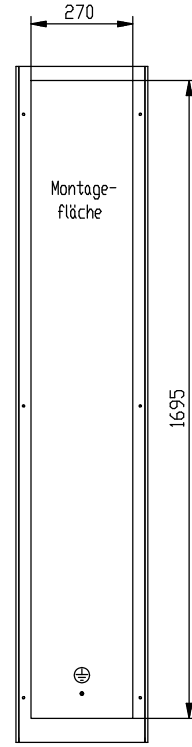
Seitenwand
