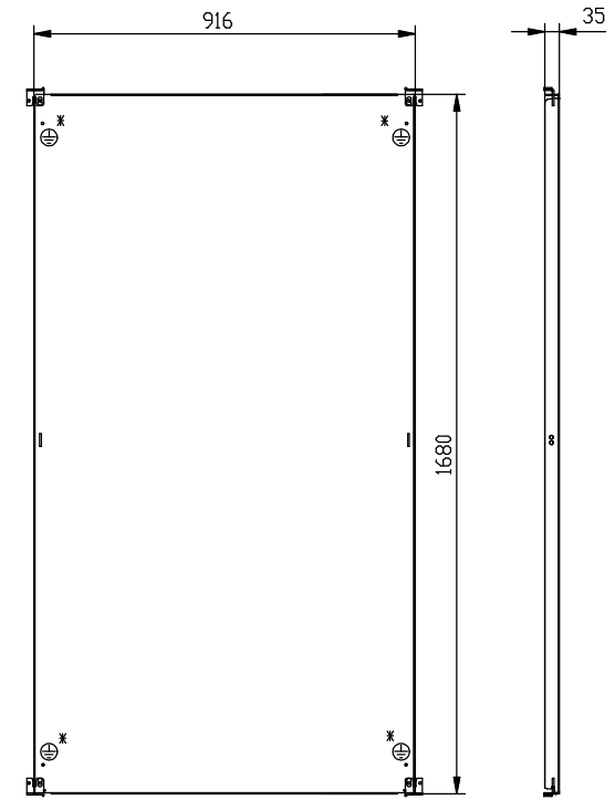
Montageplatte sendzimirverzinkt Blechstärke: 3,0 mm
