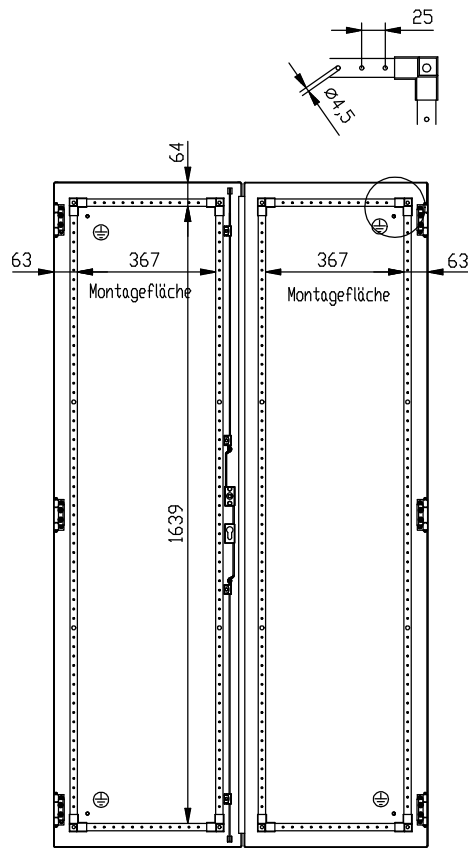
Türe Innenseite
