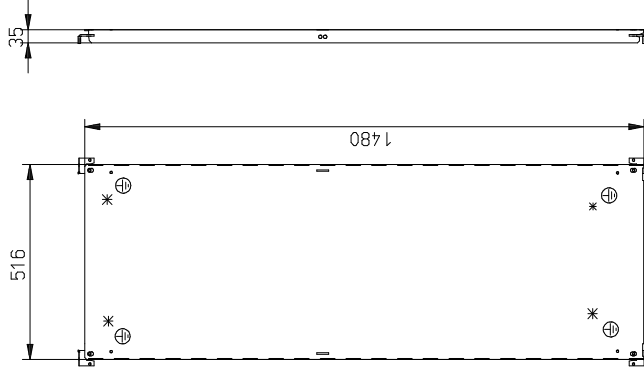
Montageplatte sendzimirverzinkt Blechstärke = 2,5 mm
