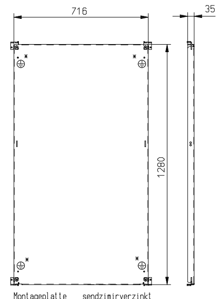
Montageplatte sendzimirverzinkt Blechstärke: 2,5 mm
