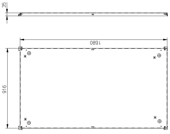
Montageplatte sendzimirverzinkt Blechstärke = 3,0 mm
