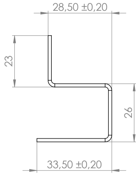
DETAIL A MAßSTAB 1 : 1
